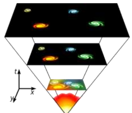
Fig: Big bang model
