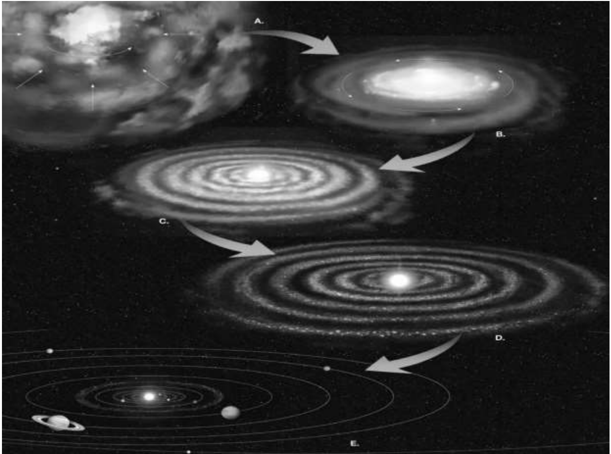
Fig: Solar Nebula
