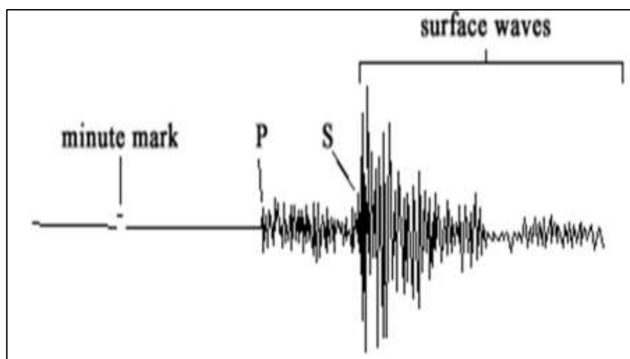
Fig: Seismogram (not seismograph)
